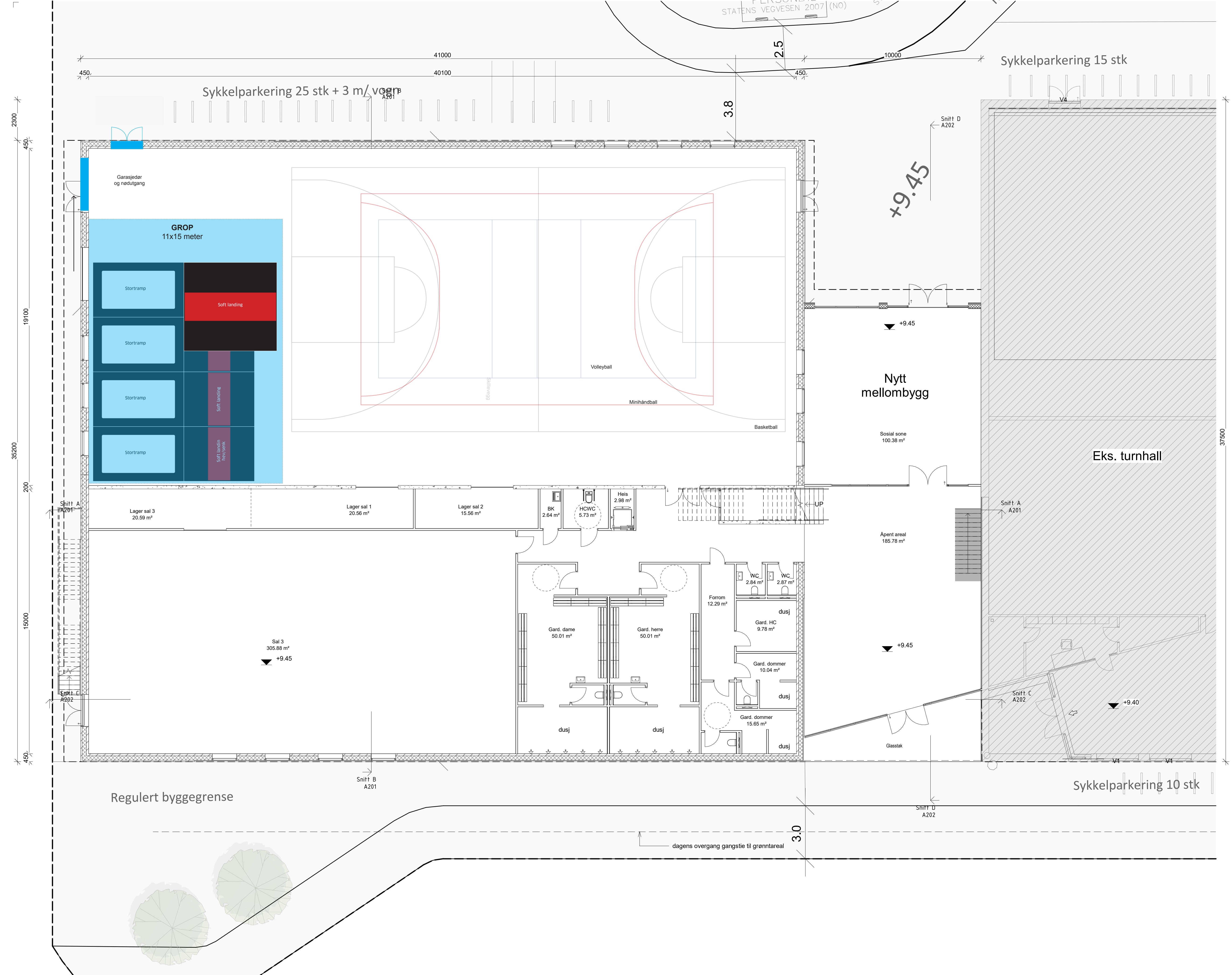
Plan 01 eks. 1 : 100
