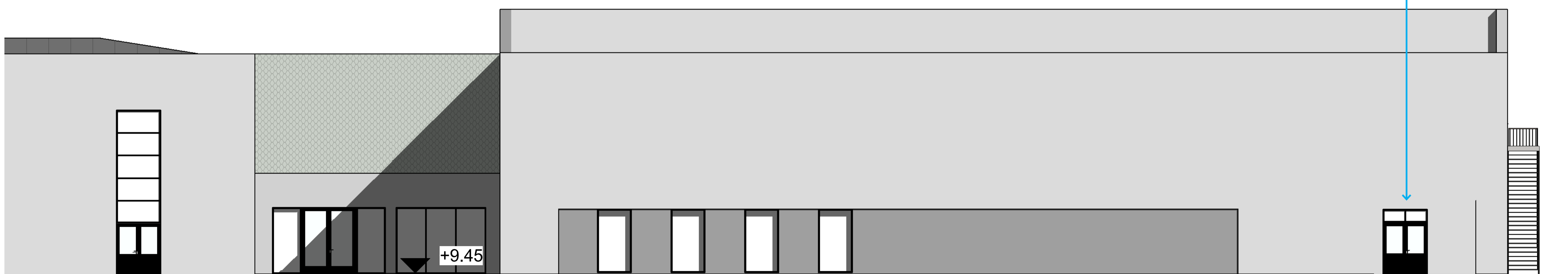
Fasade Nord-Øst 1 : 200
